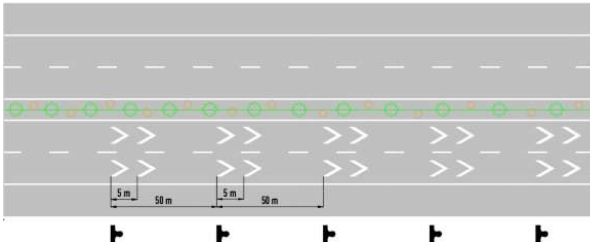
Hình G.57 - Bố trí vạch xác định khoảng cách xe trên đường
