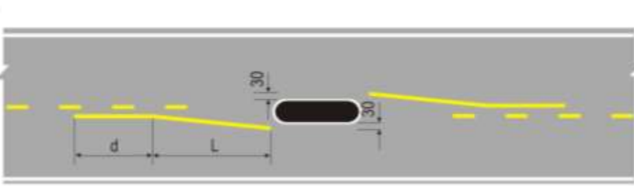
Hình G.24 - Bố trí vạch sơn cho đường hai làn xe, hai chiều xe chạy khi có chướng ngại vật nằm ở giữa đường
